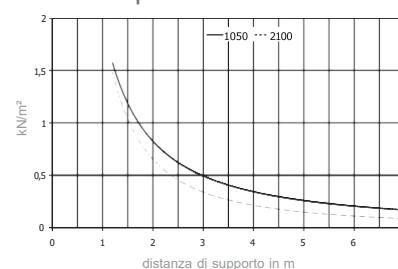
Grafico di portata
